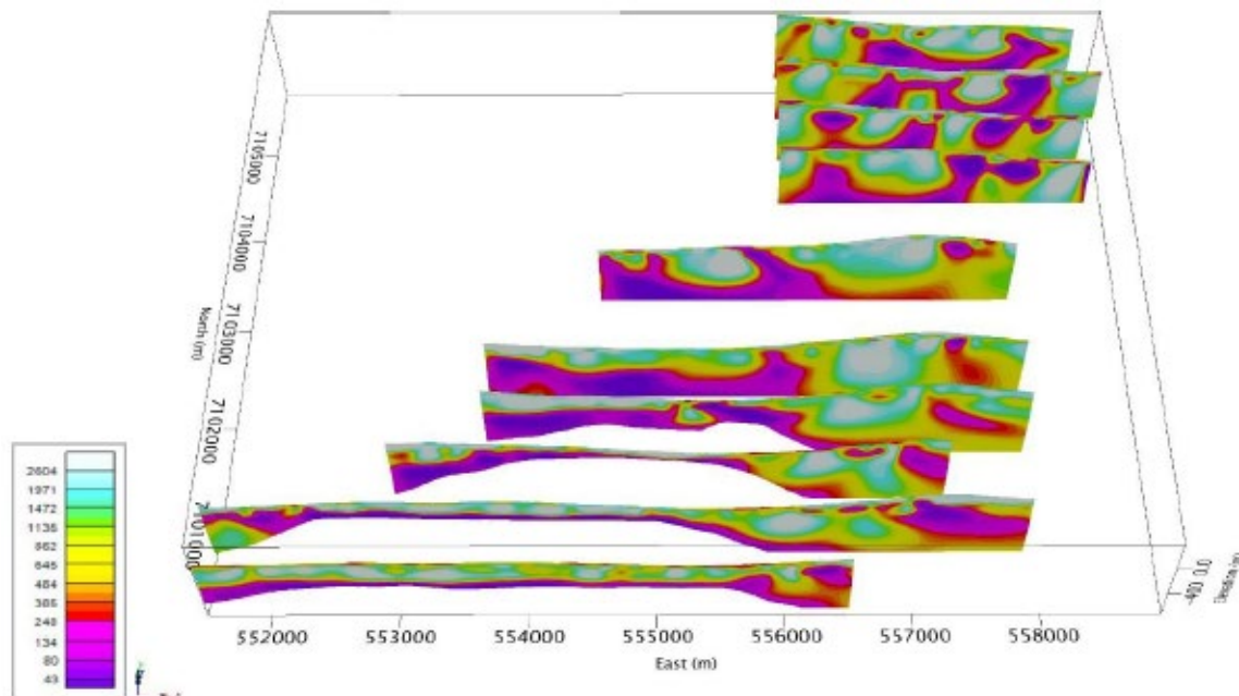
Figure 9.12: 2022 CSAMT Survey
